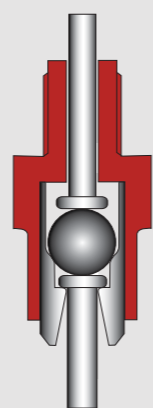
360 Nippel mit Kugel
